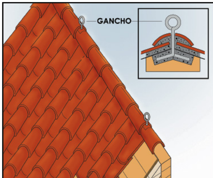
-Dibujo 2- Colocación de gancho de servicio en la cumbre de una cubierta (en esta visualización se ha decidido omitir la representación de la capa de compresión).
